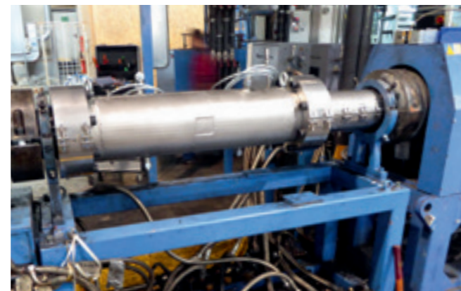
P1-Kühlmischer installiert in XPS-Dämm- plattenanlage
